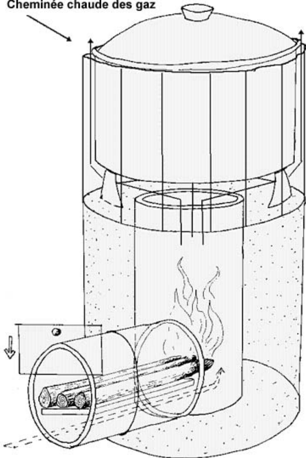
Cheminée chaude des gaz
